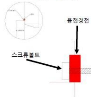
<고정부1 확대도면>
