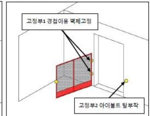
<EV 안전 난간대 설치 후 경첩을 이용한 여닫이 예시>
