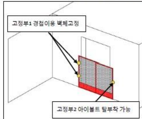
<EV 안전 난간대 설치 후 경첩을 이용한 여닫이 예시>
